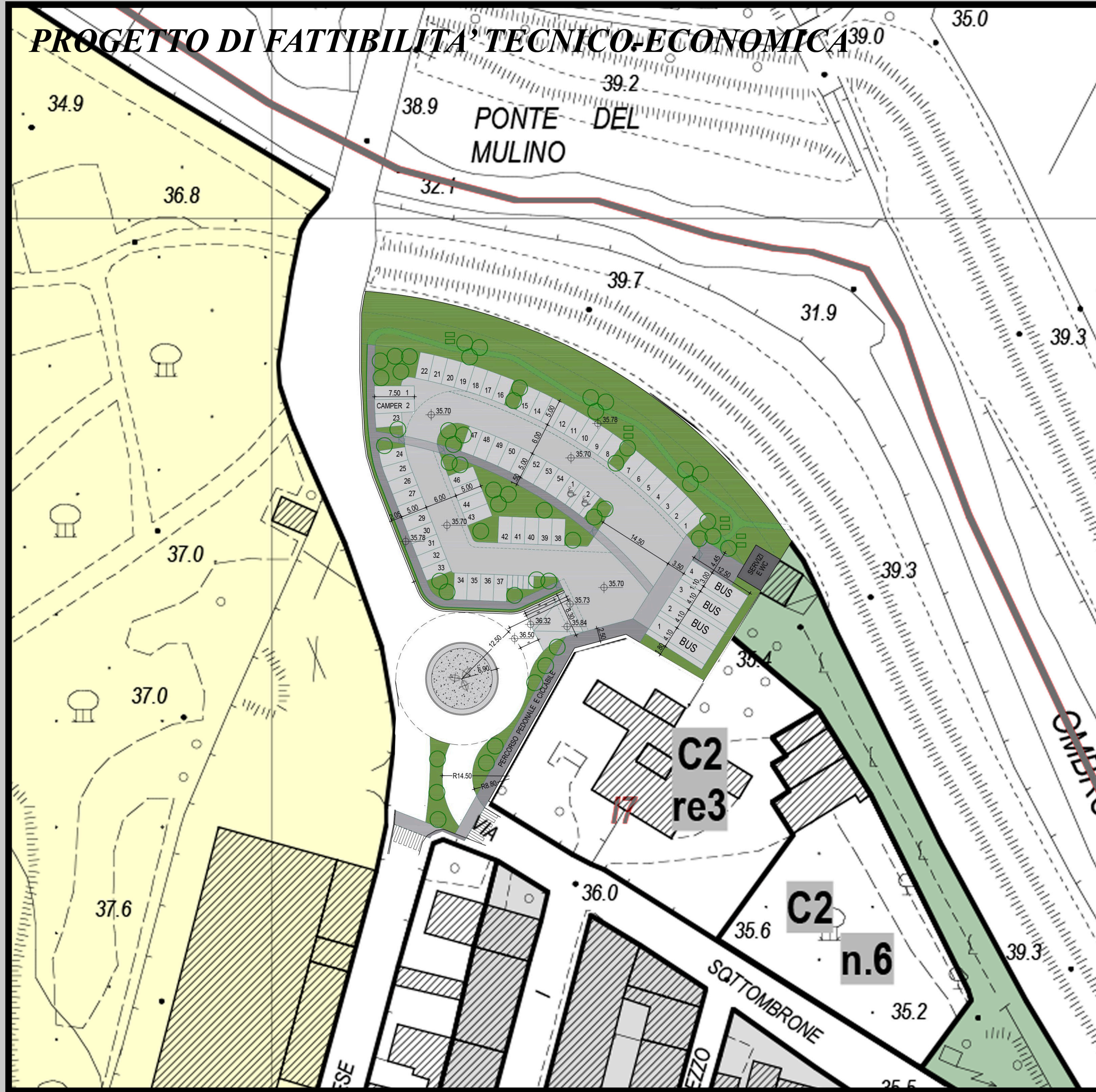
PROGETTO PRELIMINARE PARCHEGGIO PUBBLICO E NUOVA ROTATORIA
